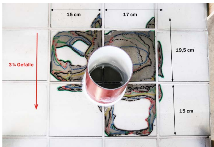
Abbildung 2: Erster Versuch – nach 72 Stunden (Buttering and Floating): Wasser, das durch die beschädigte Fuge in den Fliesenmörtel eingedrungen ist, verteilt sich diffus – völlig unabhängig vom Gefälle. Es ist in diesem Fall sogar mehr Wasser Gefälleaufwärts „gewandert“ als mit dem Gefälle. Hier liegt ein dreiprozentiges Gefälle zur Bildunterseite an, die Fliesen wurden im Buttering-and-Floating Verfahren verlegt. 42 ml der ursprünglich ca. 200 ml Wasser wurden vom Fliesenmörtel aufgenommen.
